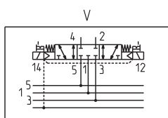
V = 5/3 лін./поз. із закритим центром
