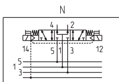
N = 5/3 лін./поз. із відкритим центром – наповнення
