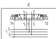
K = 5/3 лін./поз. із відкритим центром
