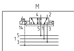
M = 5/2 лін./поз., моностабільний
