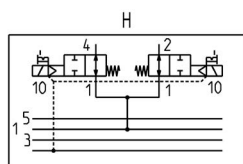
H = 2x2/2 лін./поз. Н.В.
