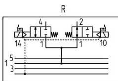
R = 1x2/2 лін./поз. Н.З. + 1x2/2 лін./поз. Н.В.
