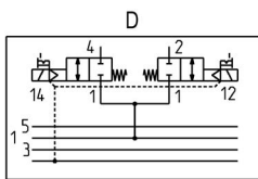
D = 2x2/2 лін./поз. Н.З.
