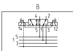
B = 5/2 лін./поз., бістабільний
