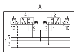
A = 2x3/2 лін./поз. Н.В.
